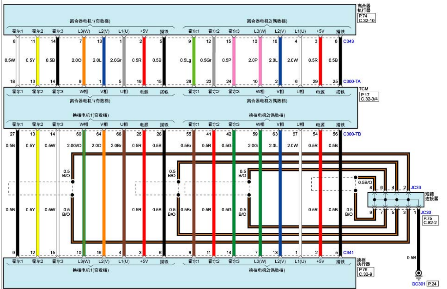
双离合变速器控制系统(G4FJ : GAMMA 1.6L T-GDI) (3)
